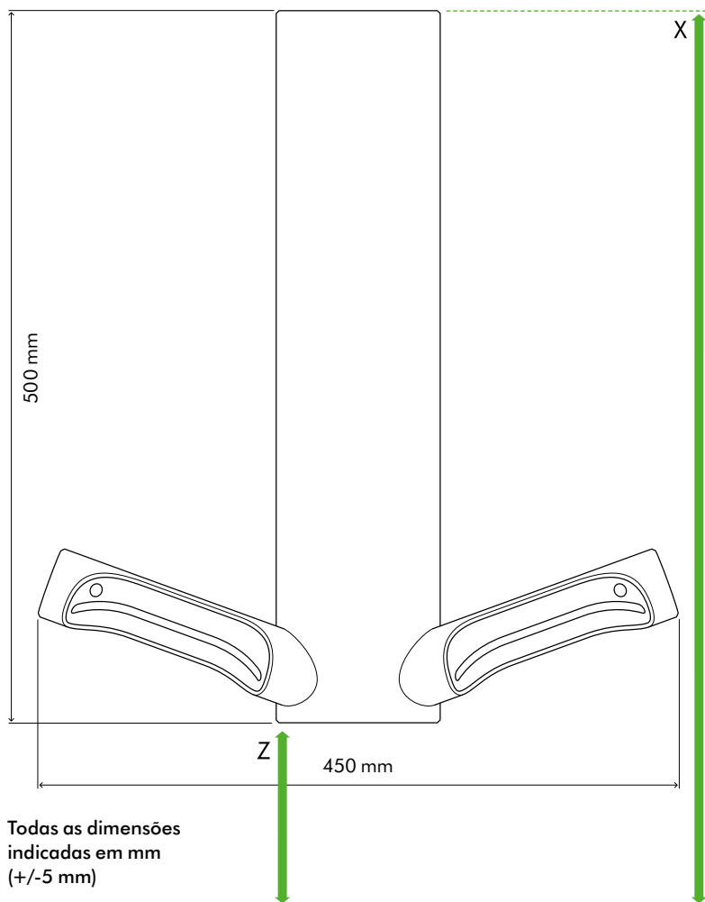
Elevação frontal
