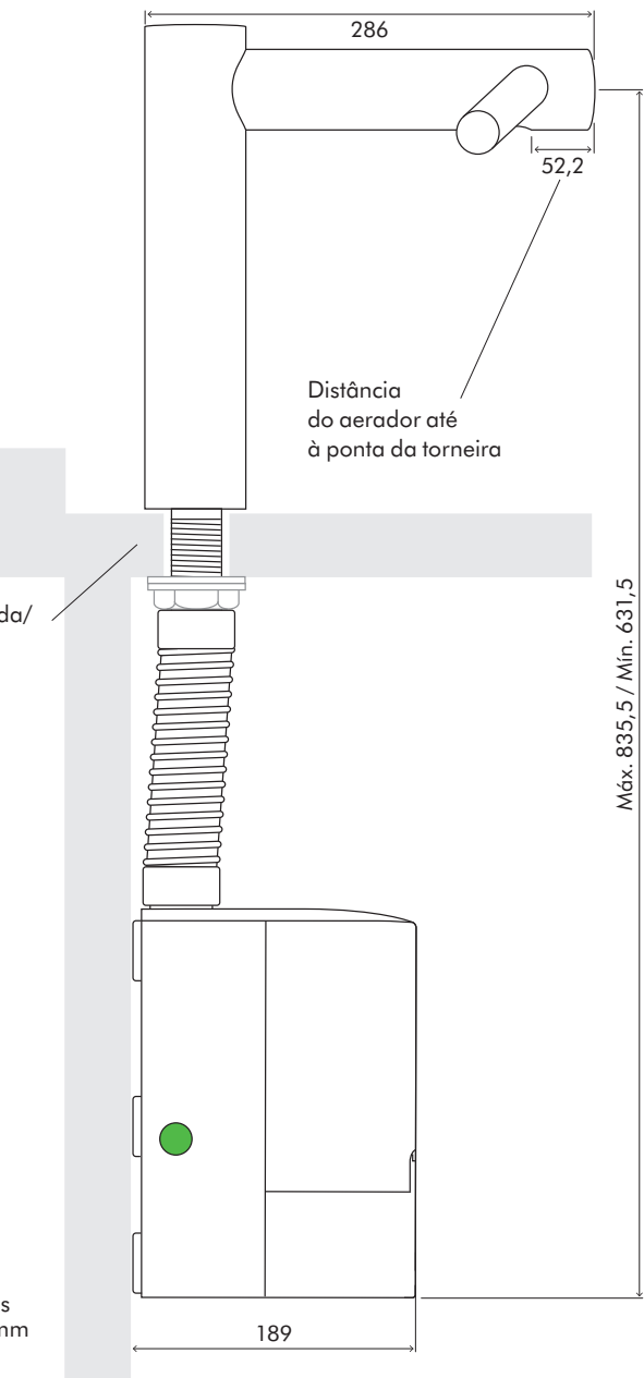
ELEVAÇÃO LATERAL
