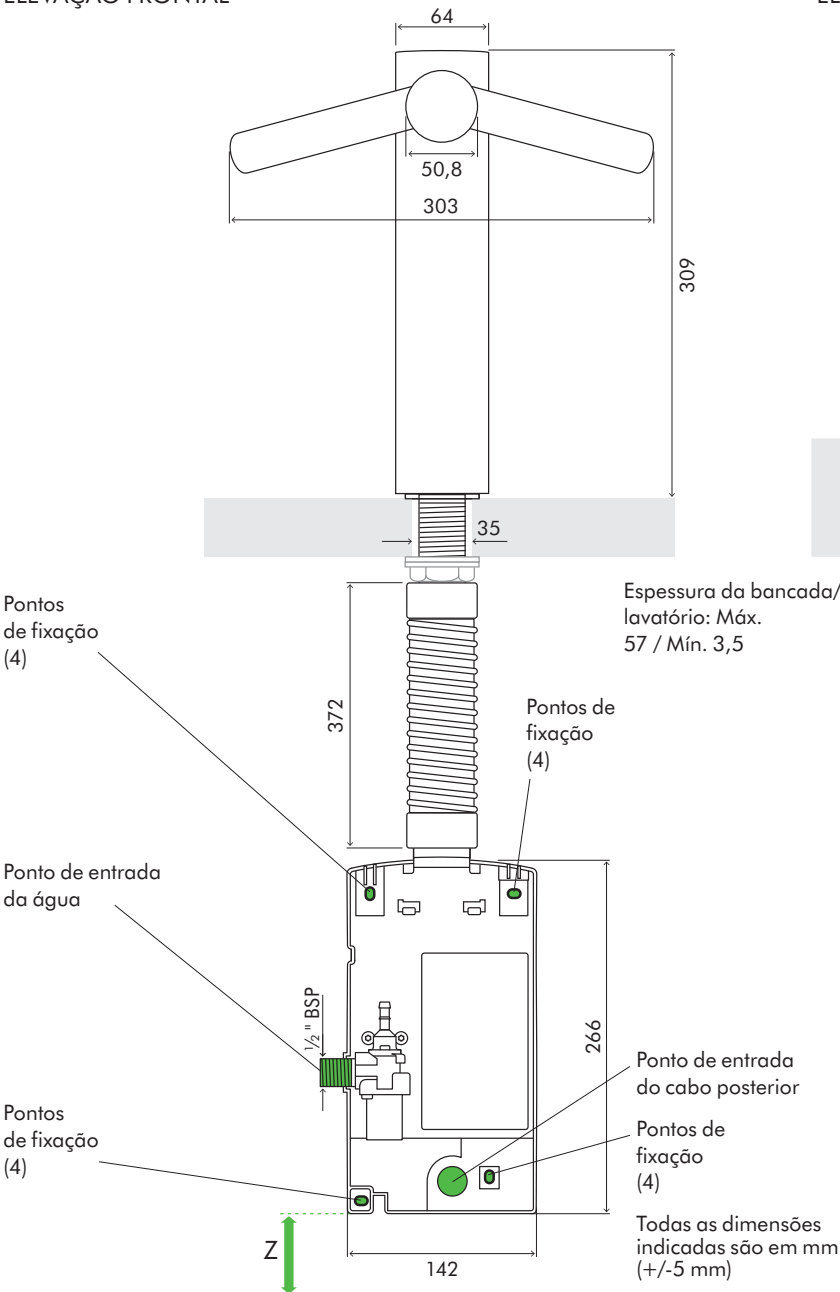
ELEVAÇÃO FRONTAL
